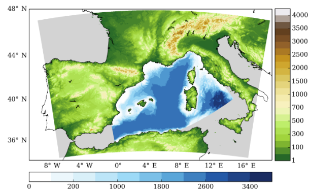
(d) MESONH-Symphonie
