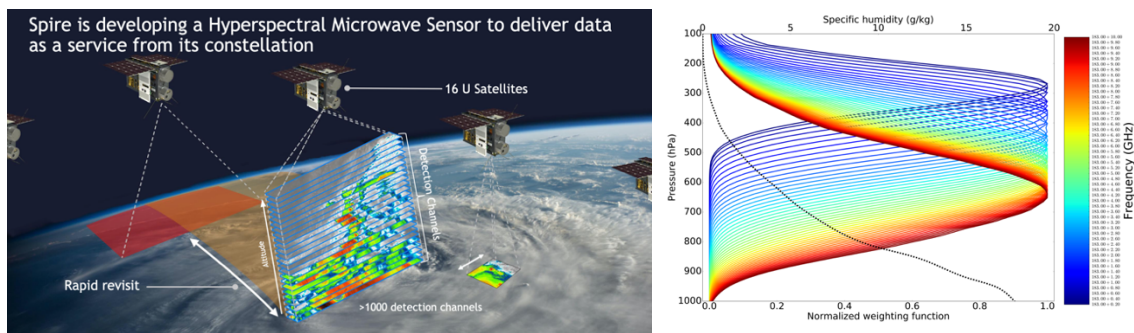
Figure 43 : (Gauche) Illustration de la future constellation d'instruments micro-ondes hyperspectraux prévue par la société américaine Spire. (Droite) Illustration de la sensibilité verticale du sondage micro-ondes hyperspectral à 183,31 GHz. La technologie hyperspectrale permet d'obtenir plusieurs milliers de canaux dans une bande d'absorption donnée, au prix d'un bruit élevé sur les mesures. Ici, un compromis entre nombre d'observations et bruit instrumental est représenté avec une soixantaine de canaux représentés alors que le nombre typique de canaux dans cette bande d'absorption de la vapeur d'eau est de 6 maximum. Source : DESR/CNRM/GMAP.
