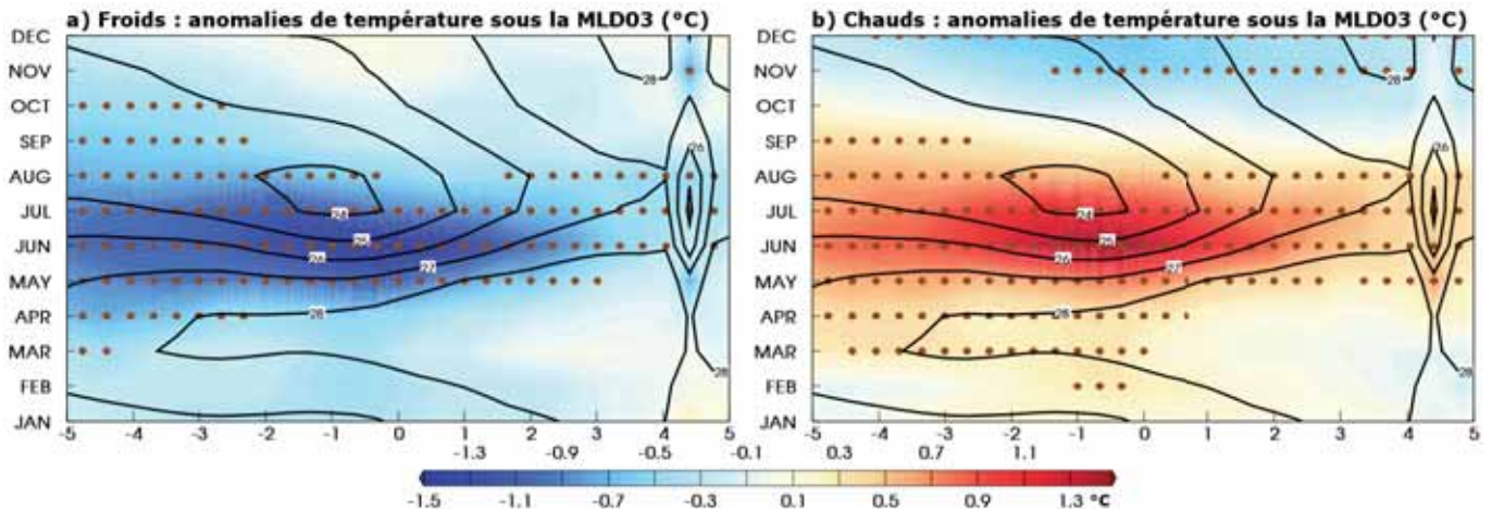
Figure 5.13 : Idem Figure 5.9 pour la température sous la couche de mélange (isolignes tous les 1°C) et les anomalies de la température sous la base de la couche de mélange (couleurs, en °C).
