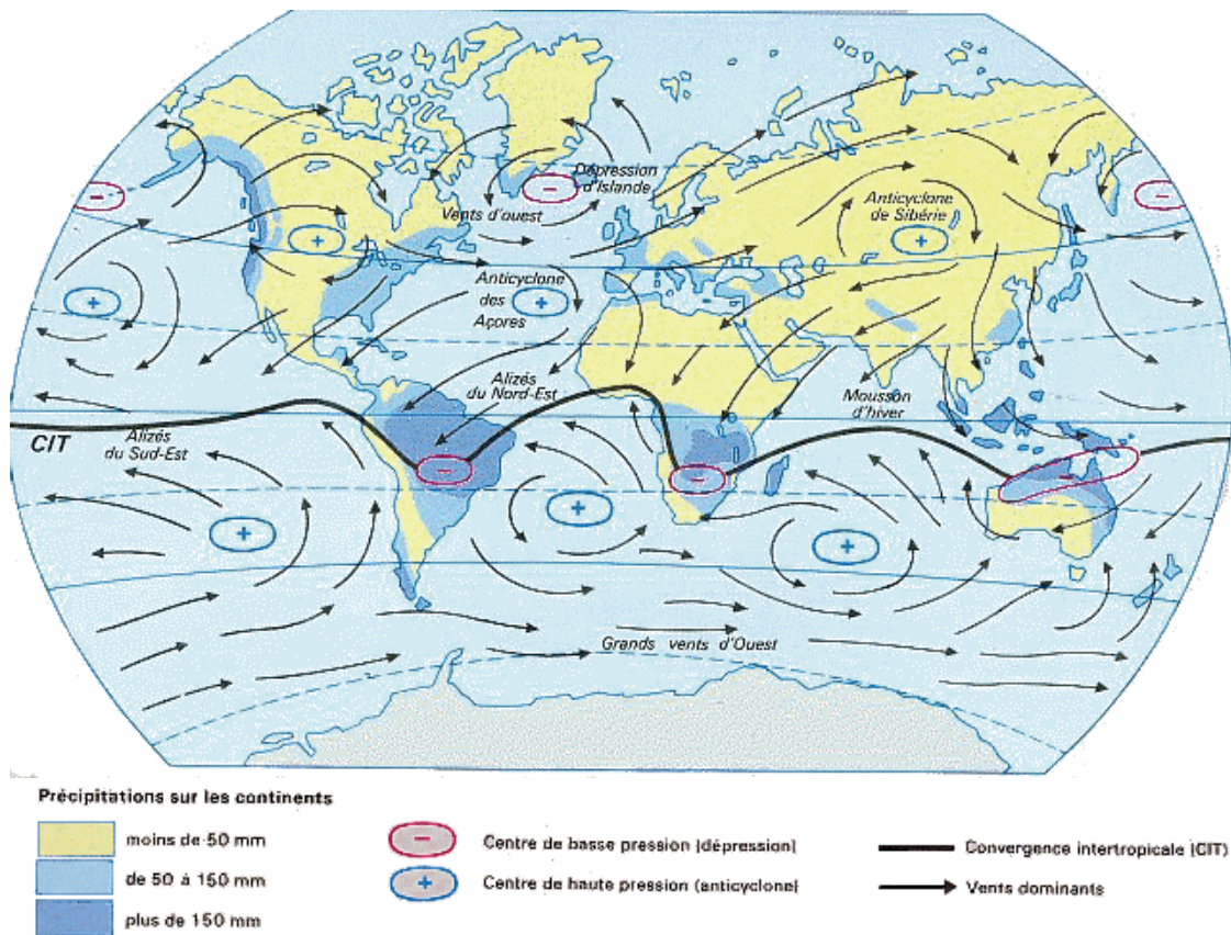
Figure 1.2 : Représentation schématisée de la circulation atmosphérique générale et des précipitations moyennes. Figure tirée de http://eduscol.education.fr/obter/applied/circula/theme/atmo322.htm .
