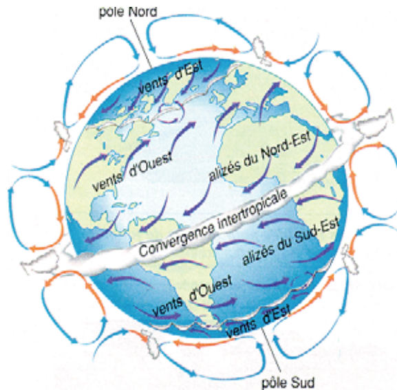
Figure 1.1 : Représentation schématisée de la circulation de Hadley. Figure tirée de http://eduscol.education.fr/obter/applied/circula/theme/atmo322.htm .
