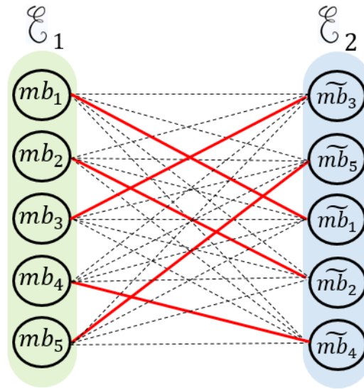
FIGURE 2.18 – Exemple d’un problème d’affectation sous forme de graphe biparti. L’objectif de l’algorithme de Munkres est de trouver une bijection entre les membres des deux ensembles \mathcal{E}_1 et \mathcal{E}_2 , avec une distance totale d’affectation (somme des arêtes rouges dans cet exemple) minimale.
