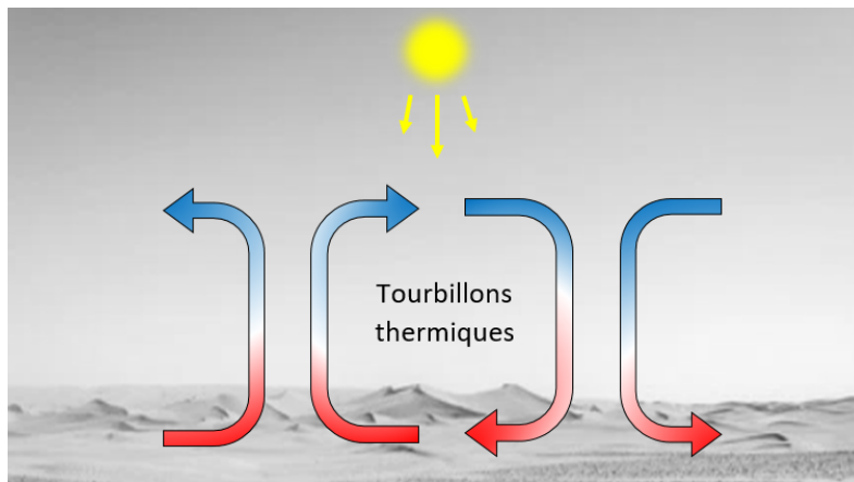
FIGURE 1.3 – Représentation schématique de la turbulence d’origine thermique, et la création des gros tourbillons thermiques. Les masses d’air chaud au voisinage du sol sont représentées par la couleur rouge, alors que les masses d’air froid en altitude sont représentées par la couleur bleue.
