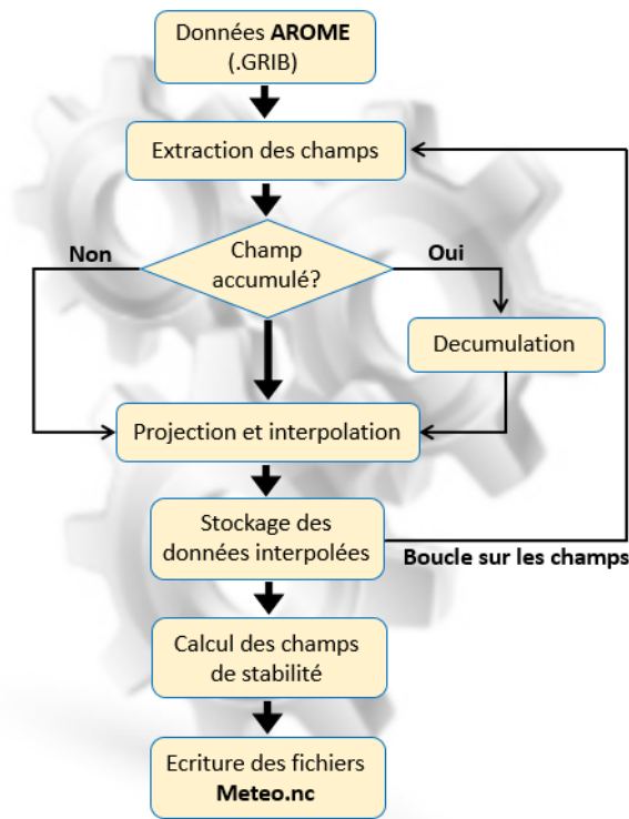
FIGURE B.1 – Organigramme décrivant l’ensemble des processus réalisés par l’algorithme AROME-to-pX dans le cadre de ces travaux de thèse. Cet algorithme, développé en langage Python (version 3.8), permet d’obtenir les données météorologiques utilisées en entrée du modèle pX (format netCDF), à partir des données en sortie d’AROME.
