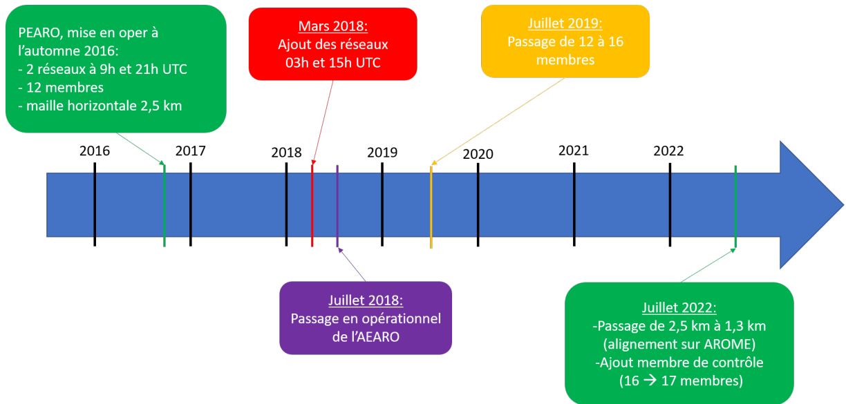
FIGURE 2.13 – Chronologie des principales évolutions de la prévision d'ensemble PEARO depuis sa mise en opérationnel pour la première fois en 2016 jusqu'au 2022. Source Mounier (2022) .
